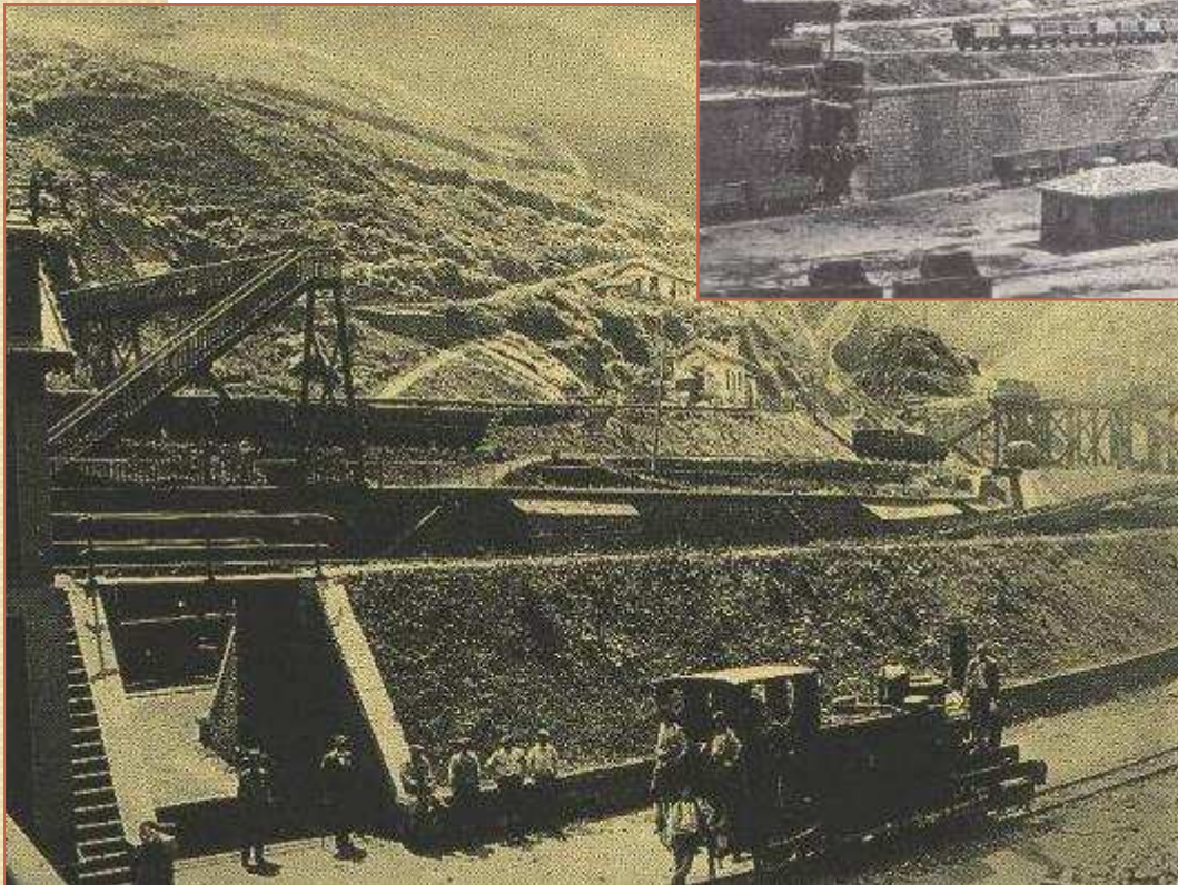
Estación de Orkonera y pie del plano inclinado (1893)
