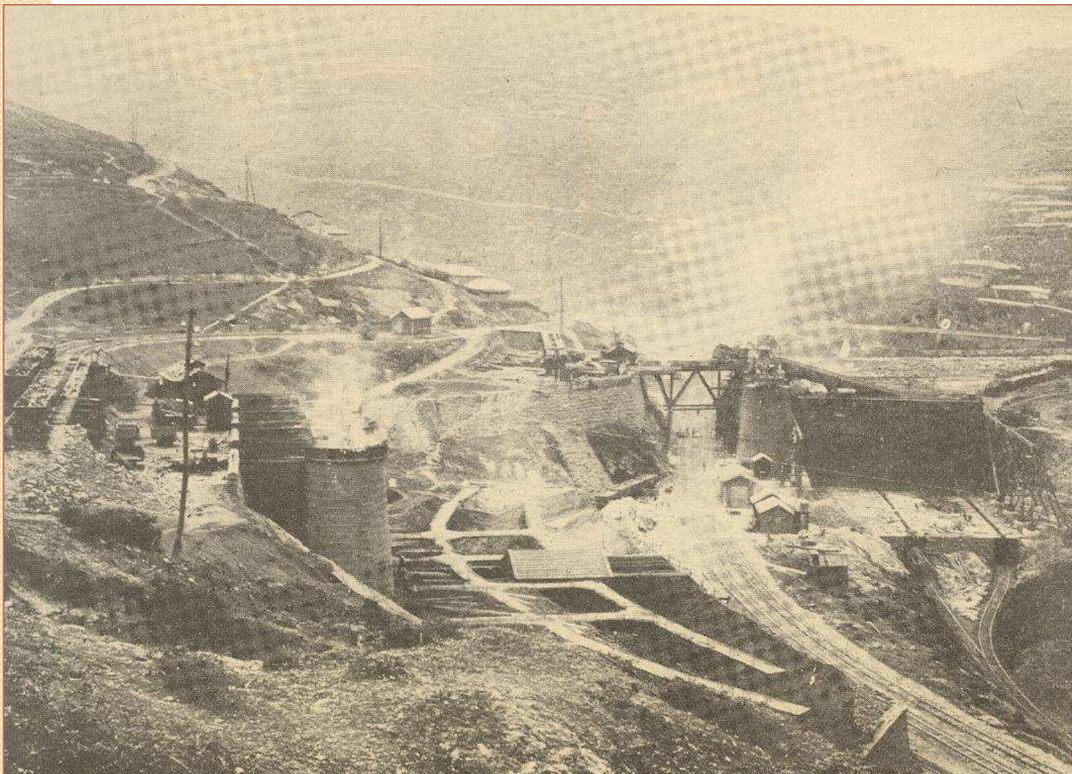
Batería de hornos de calcinación en la Estación de Orkonera
